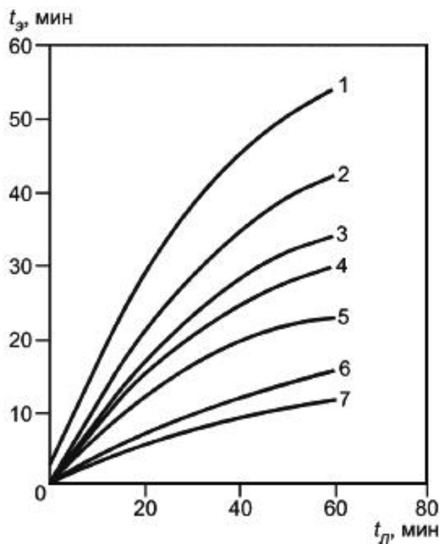
Рисунок Р.6 - Зависимость эквивалентной продолжительности пожара t_3 от продолжительности пожара t_{п} для вертикальных незащищенных металлических конструкций
